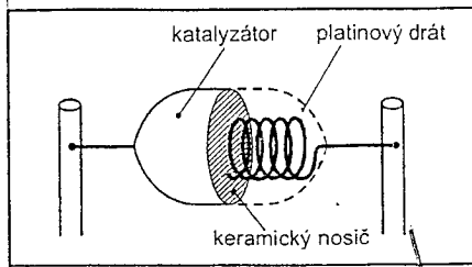
Obr. 2. Struktura pelistoru
