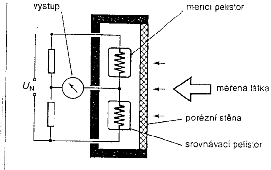
Obr. 3. Měřicí můstek s pelistorovými senzory
