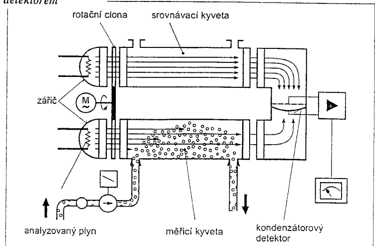
Obr. 9. IČ analyzátor s pozitivní filtrací
