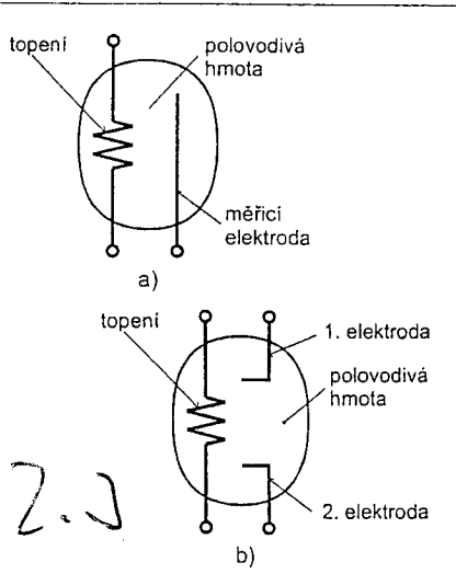
Obr. 4. Schematické uspořádání polovodiivého senzoru
