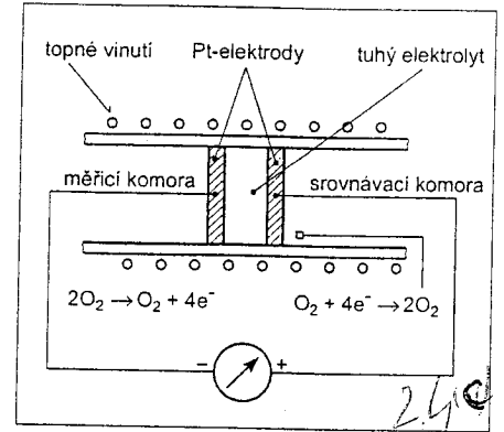
Obr. 6. Schéma elektrochemického senzoru s pevným elektrolytem
