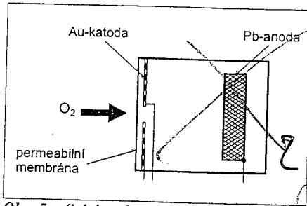
Obr. 5. Schéma kyslíkového senzoru
