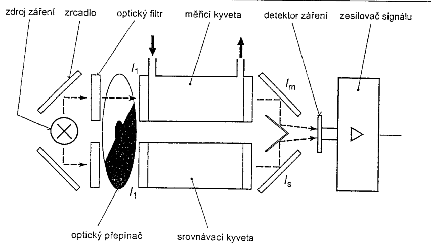
br. 8. Schéma dvoupaprskového fotometru se společným zdrojem a detektorem
