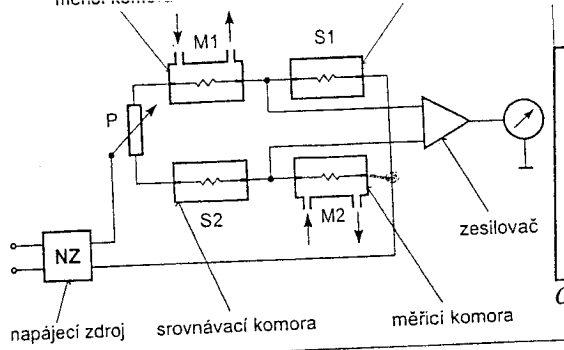
Obr. 1. Měřicí můstek tepelněvodivostního senzoru
