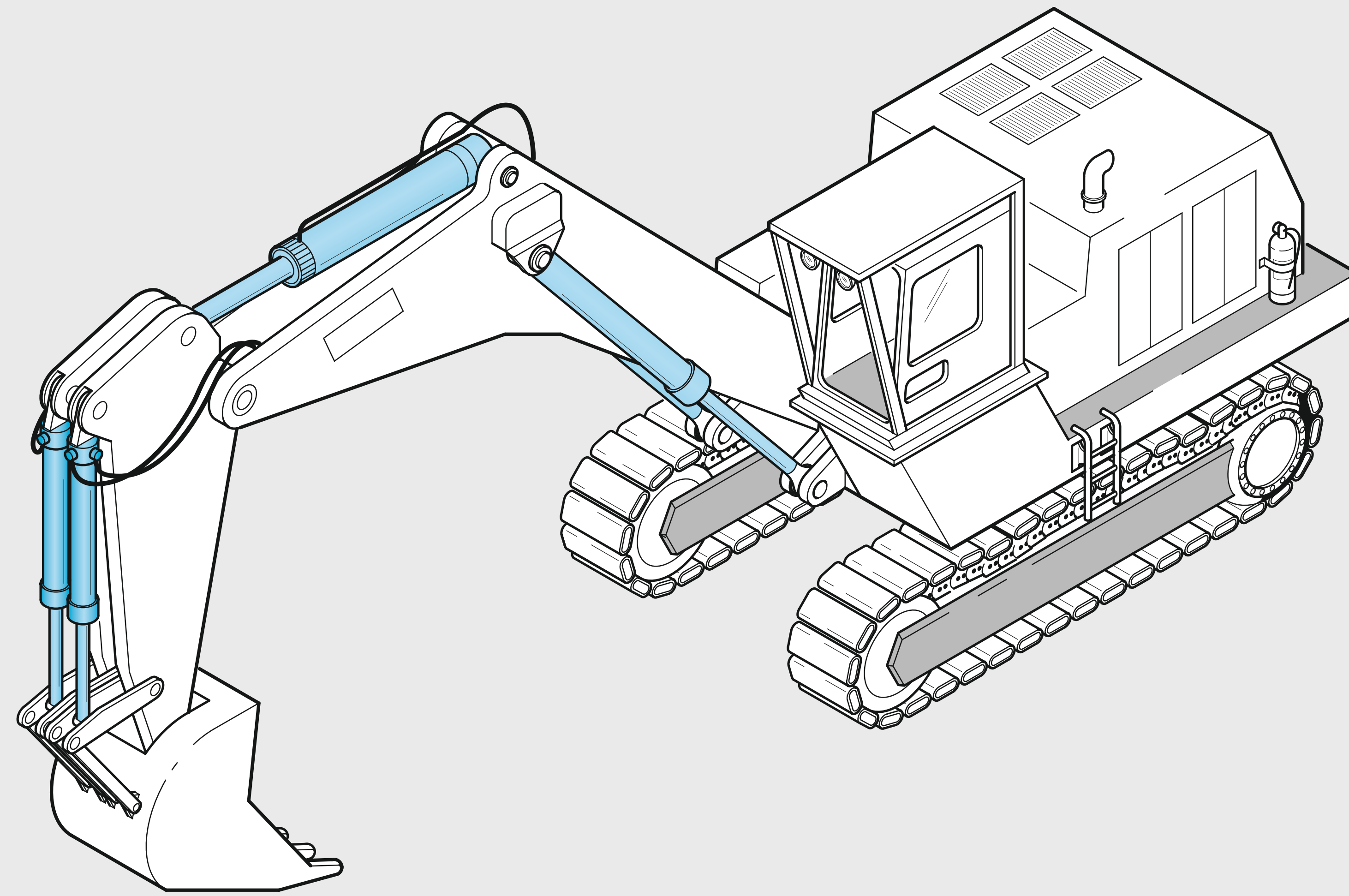
Mobilní hydraulika - příklad: bagr
